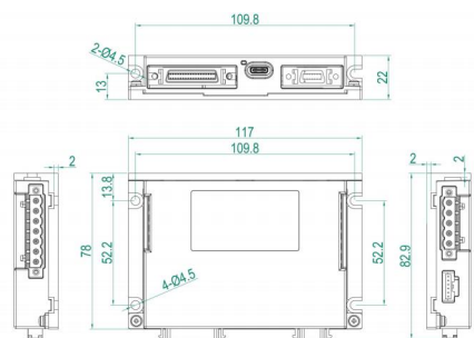
LVD2-AP/AP2 安装尺寸(单位: mm)
