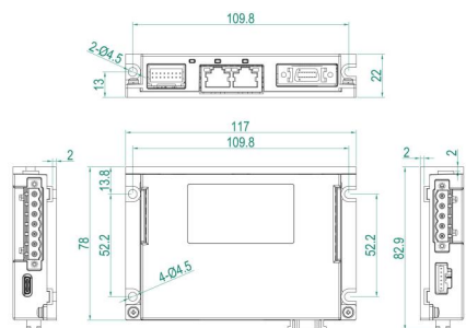
LVD2-EB/EC2 尺寸(单位: mm)
